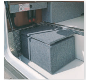
»17005« Subwoofer platzsparend installiert (im Gepäckraum / Doppelboden)
