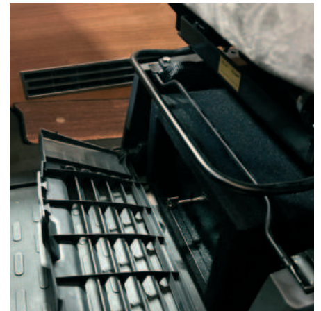
Safe'n'Sub unter dem Beifahrersitz montiert (Fiat Ducato)
